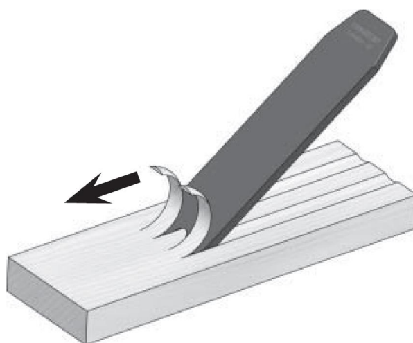
Abbildung 1: Herstellen einer Abziehform aus Holz
